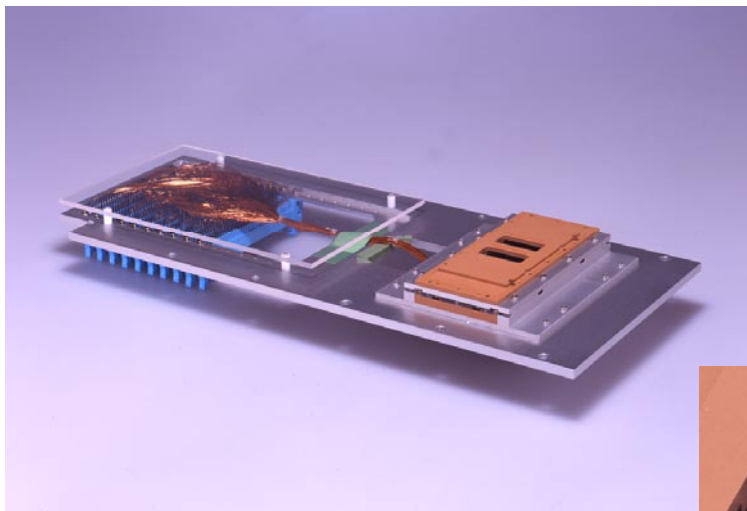
TAB / COFキャリアテープ検査用テストヘッド
