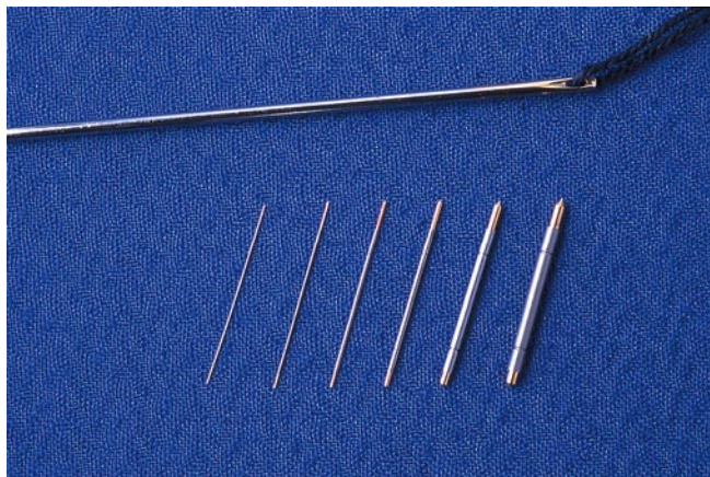
超極細コンタクトプローブ ( \phi 0.11 ～ \phi 0.72 mmコンタクトプローブ6機種)
