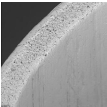
不透過マーカの内外面エッジ (バリ無し加工)
