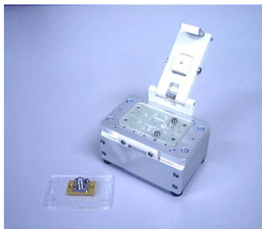
【写真】高周波モジュール用検査治具ヘッド(RFTH-10シリーズ)と測定アダプタ
