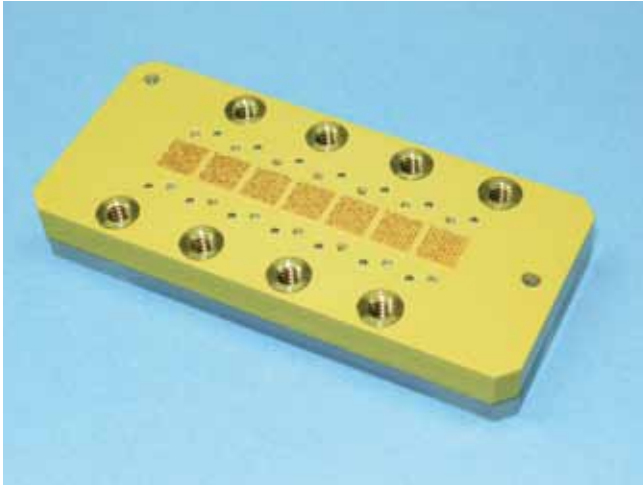
ストリップソケット
