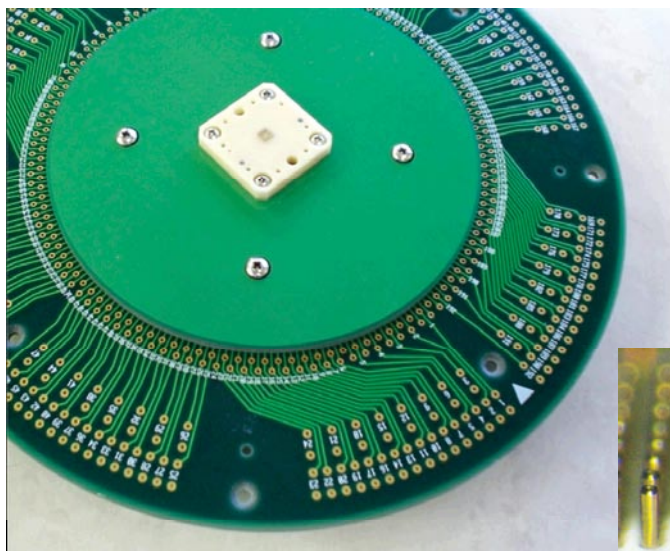
垂直型プローブカード(YVPシリーズ)
