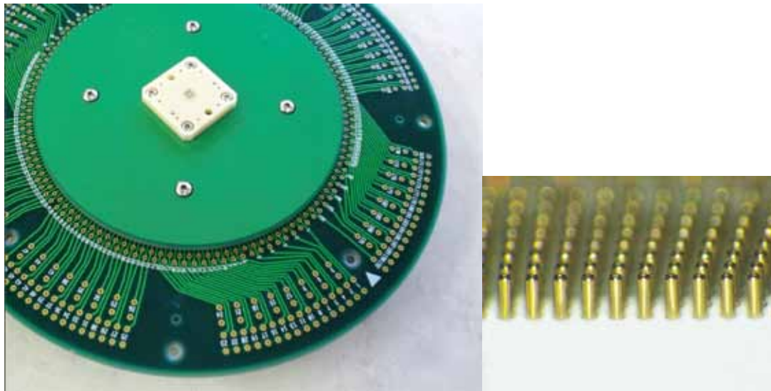
垂直型プローブカード (YVPシリーズ)
